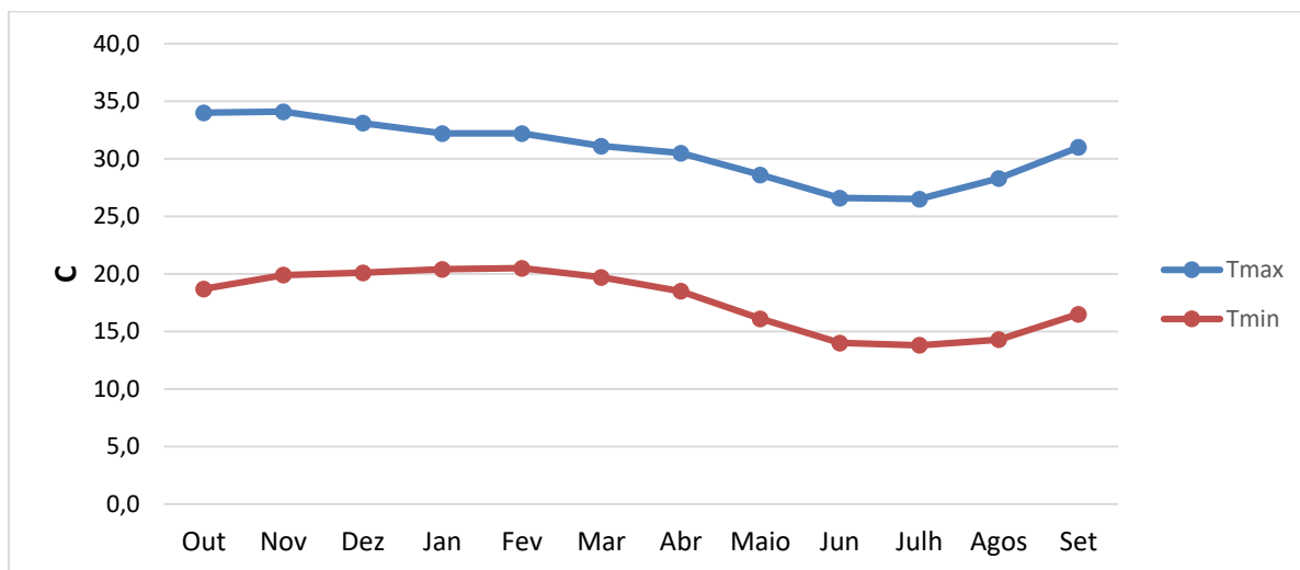
Figura 2: Padrão anual das temperaturas máximas e mínimas para a região de influência da estação de Inhaminga.
