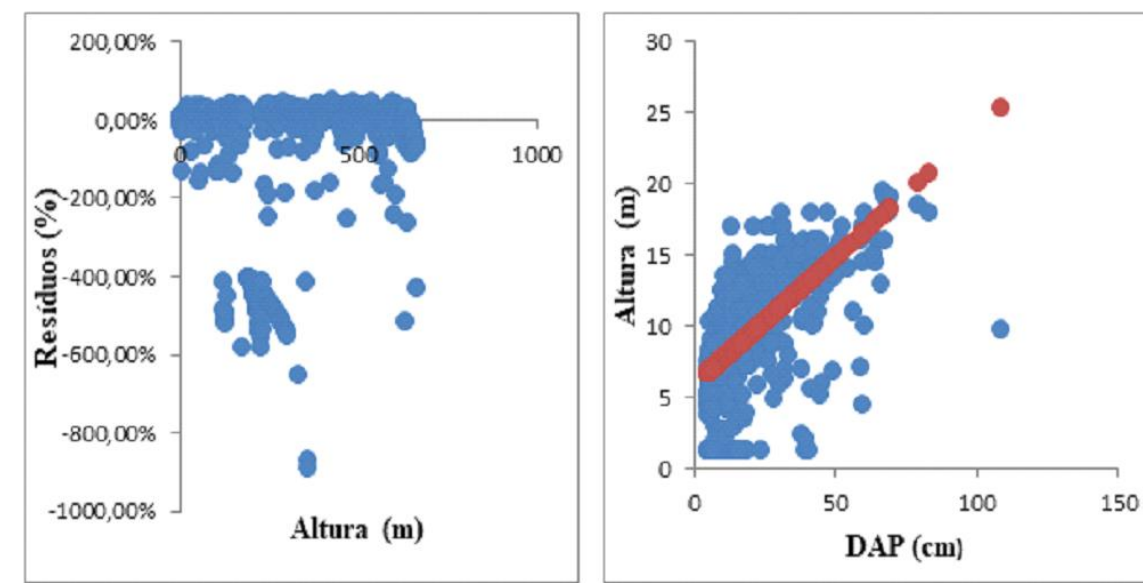
Figura 19: Gráfico de resíduos e de ajuste do modelo da Linha recta.
